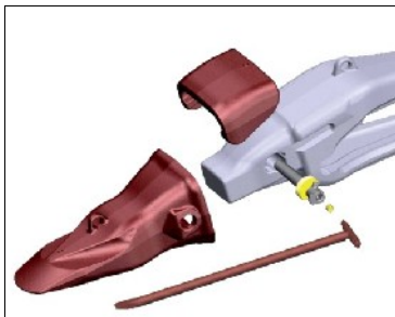
Starmet
