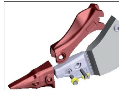
Ripmet
